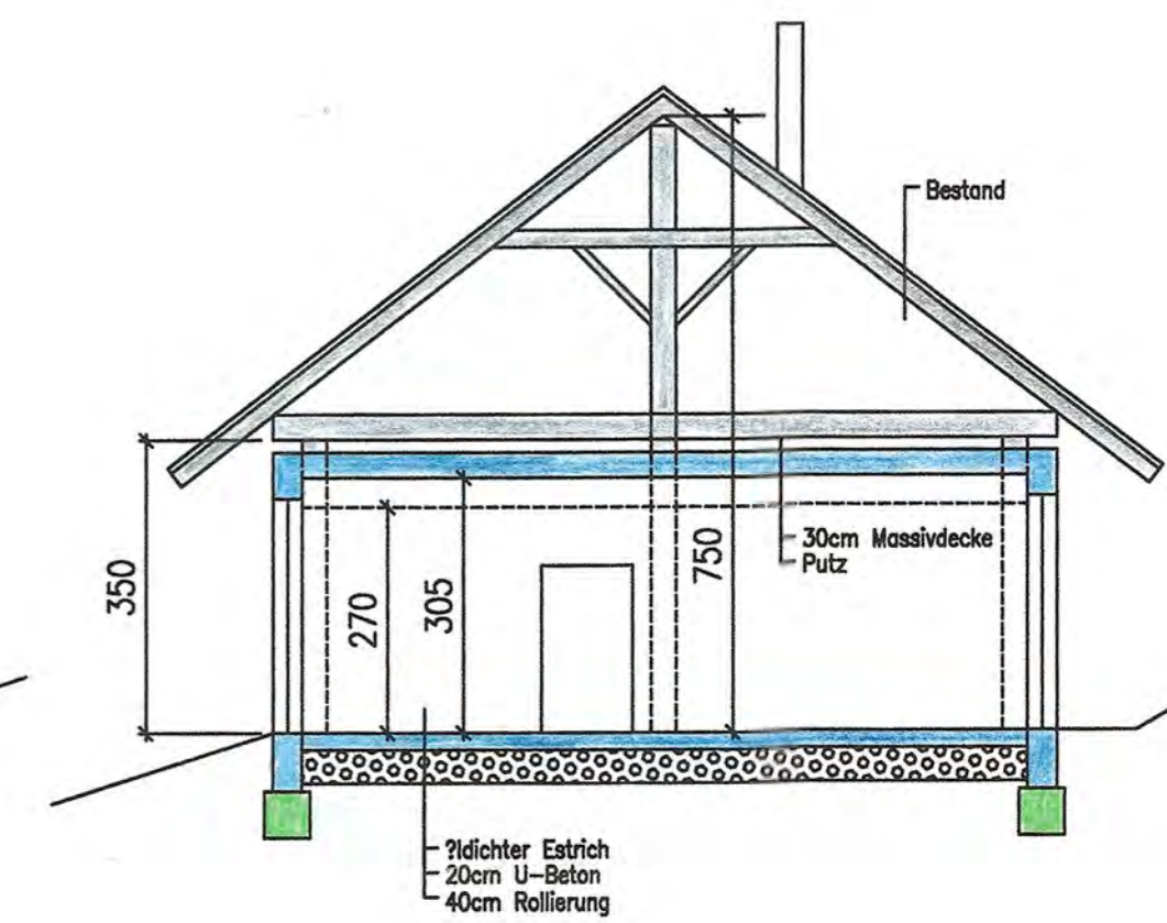
Schnitt B-B
