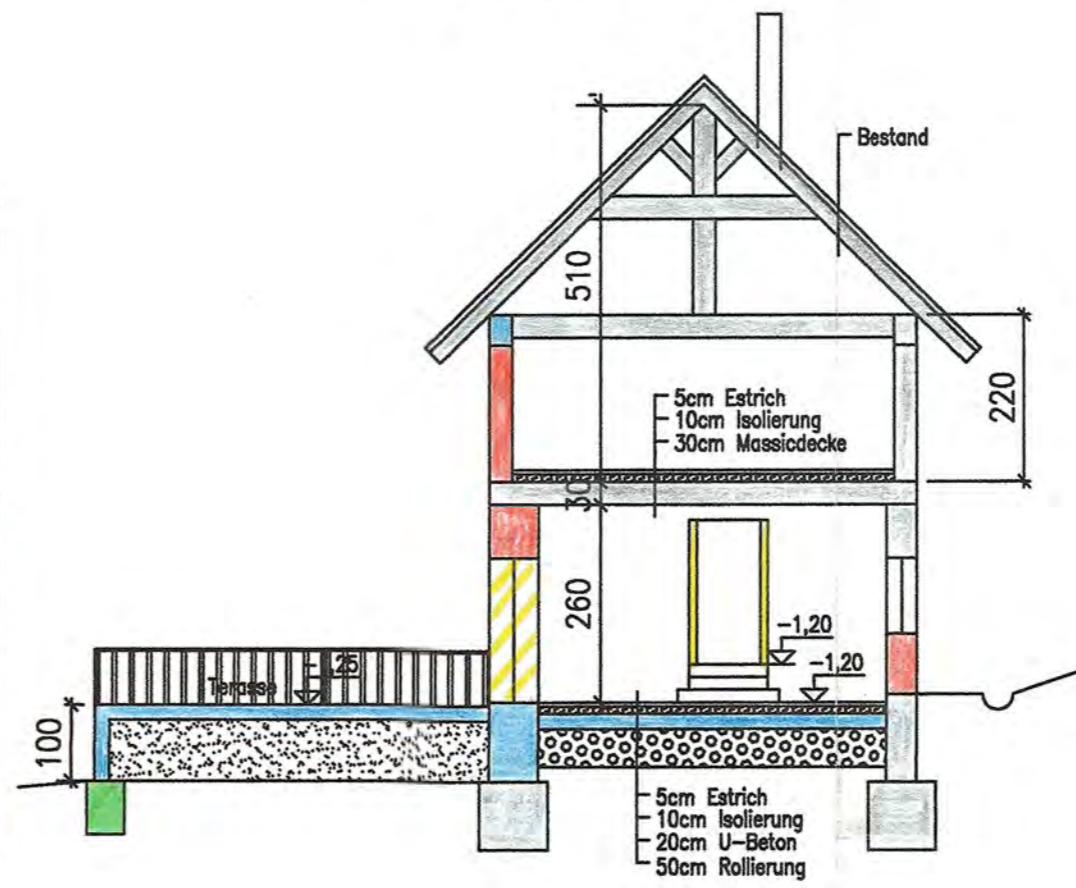
Schnitt A-A
