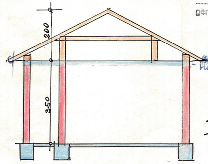
SCHNITT
